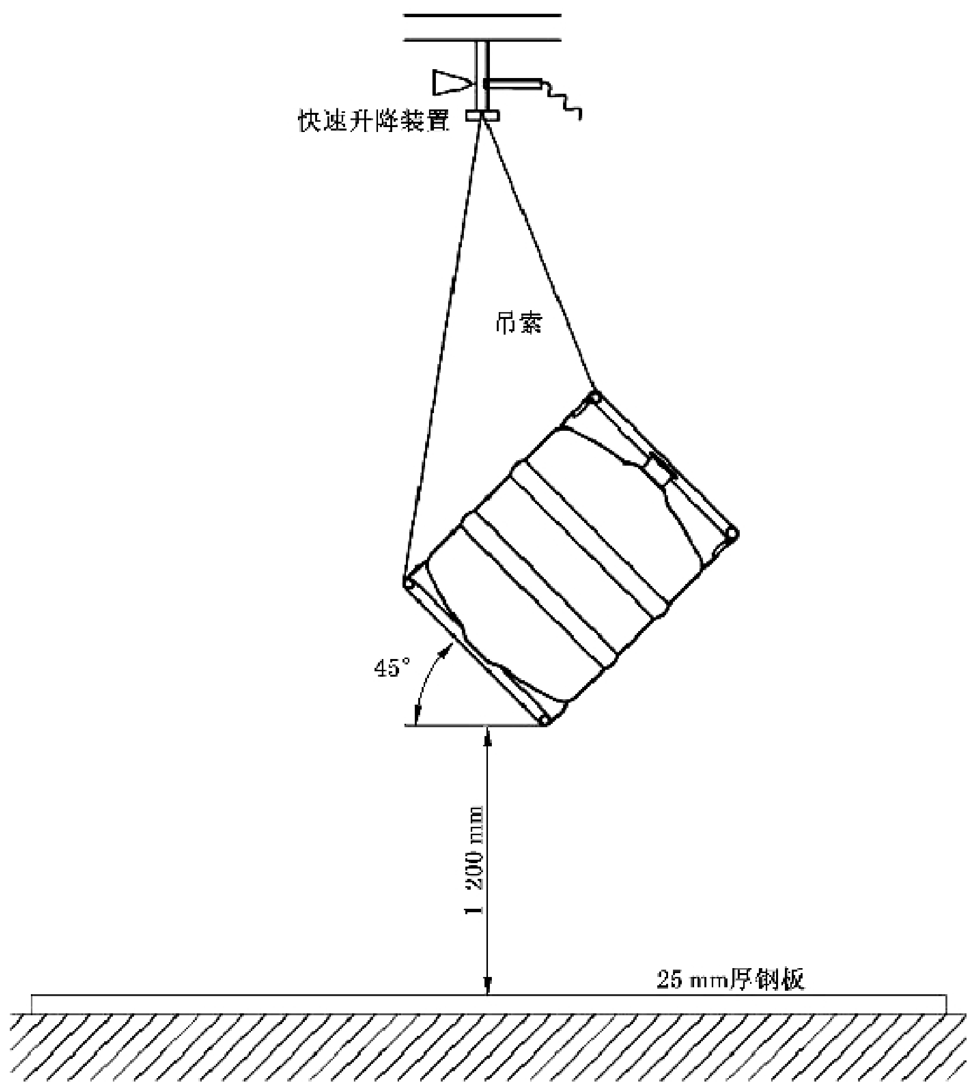
图 9 下圈成 45° 跌落试验示意图
