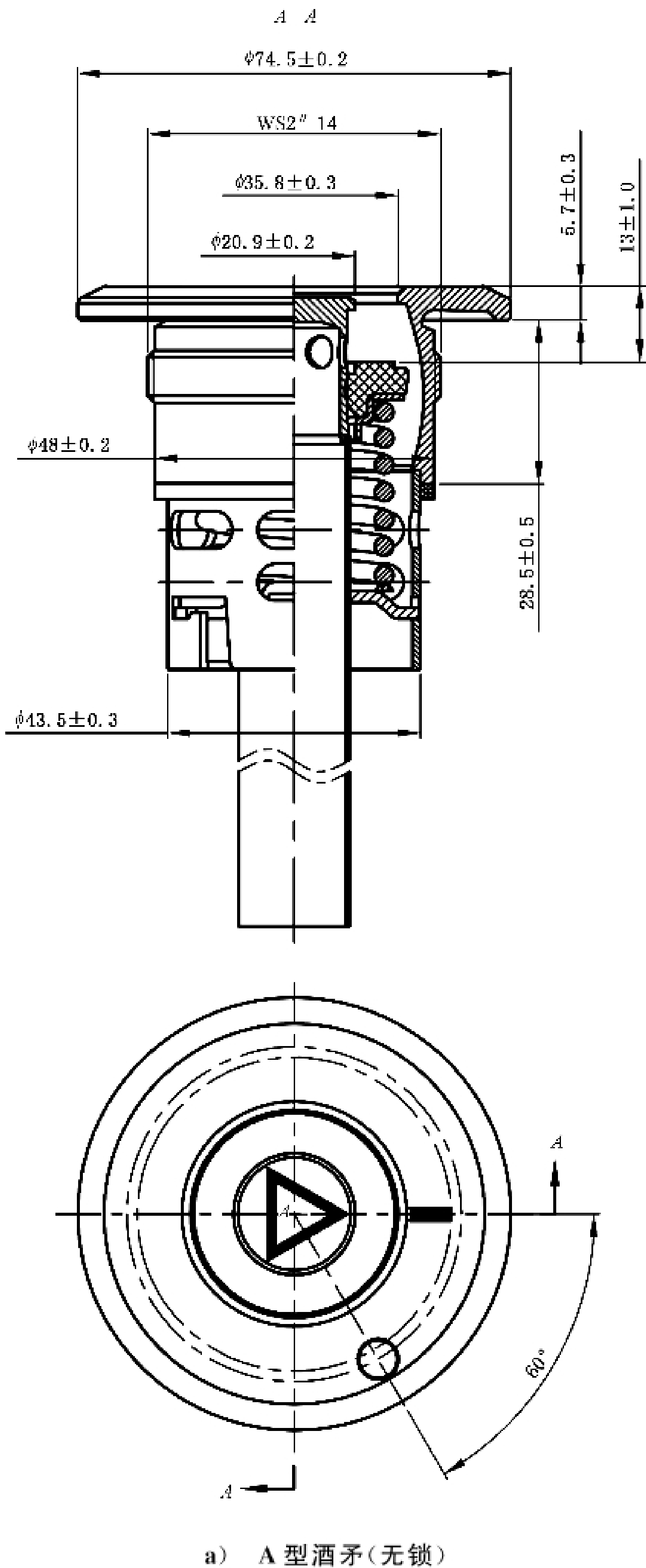
图 A.1 酒矛外形及螺纹尺寸示意图
