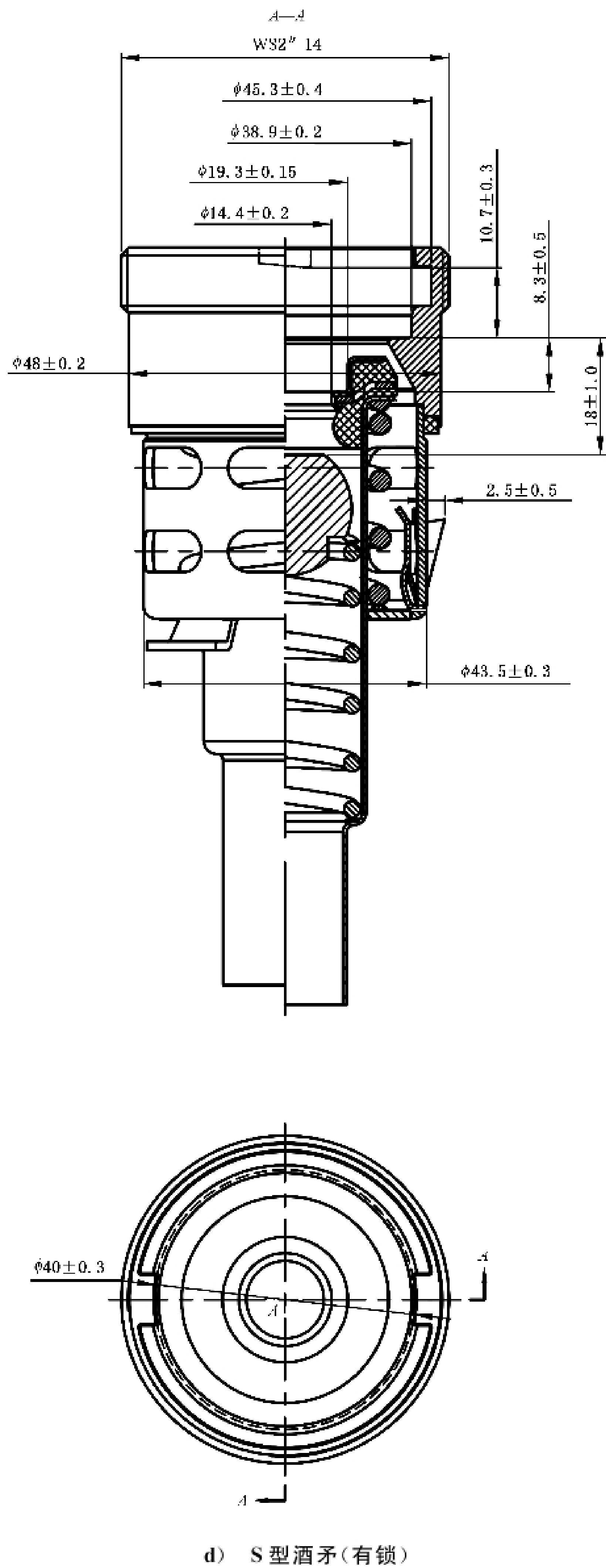
图 A.1 酒矛外形及螺纹尺寸示意图 (续)
