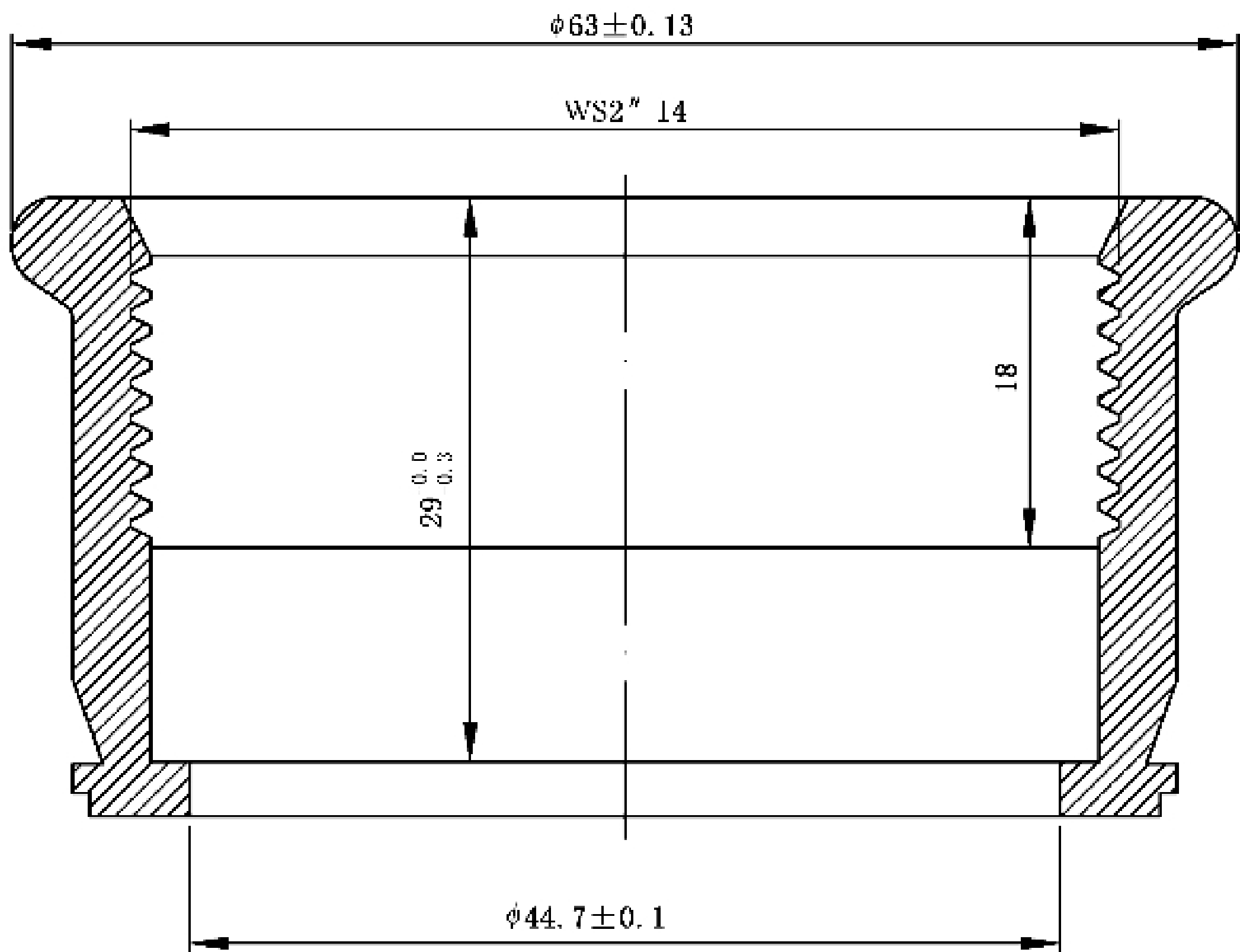
图 B.1 酒矛座外形及螺纹尺寸示意图
