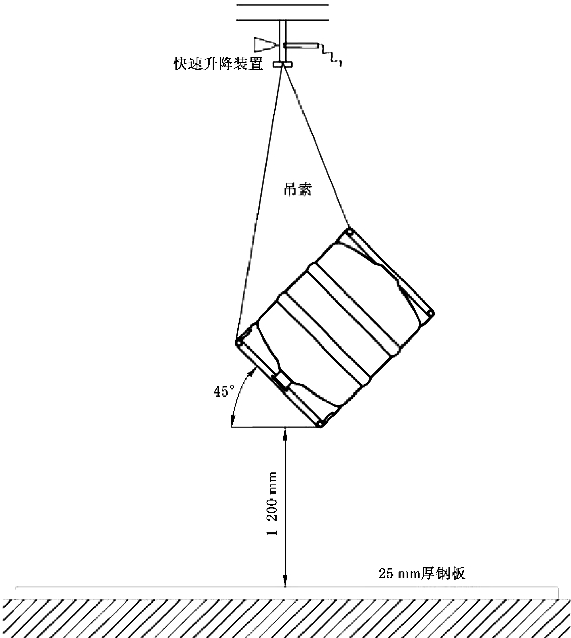
图8 上圈提手孔成45°跌落试验示意图
